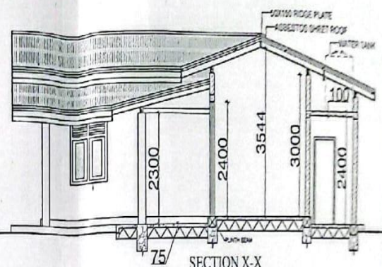
SECTION X-X SCALE: 1:100
